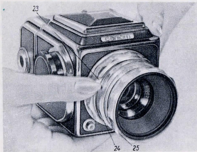
Рис. 7. Открыва- ние диафрагмы:
