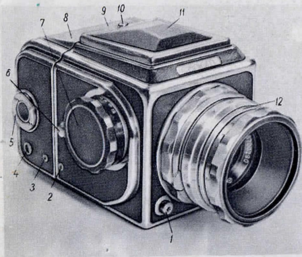
Рис. 1. Общий вид фотоаппарата «Салют»:
