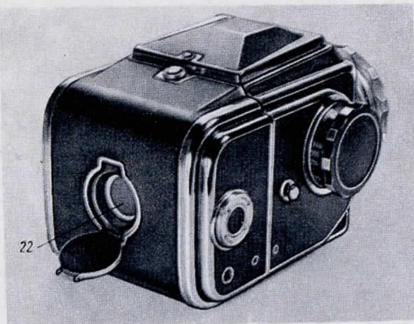
Рис. 6. Смотровое окно (22).
